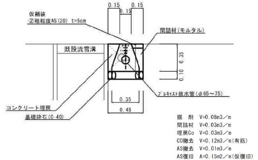
標準断面図(仮復旧) S=1:20 (流雪溝隣接部)
