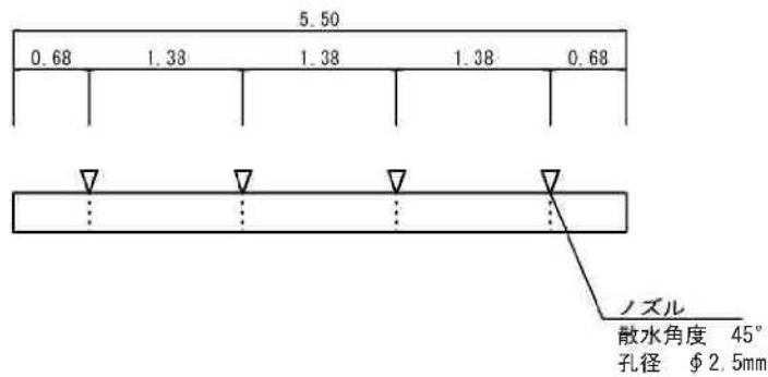
散水用ノズル位置(タイプⅡ) S=1:50
