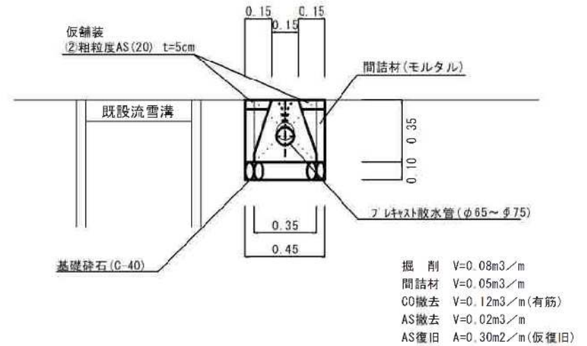
標準断面図(仮復旧) S=1:20 (神明橋側)
