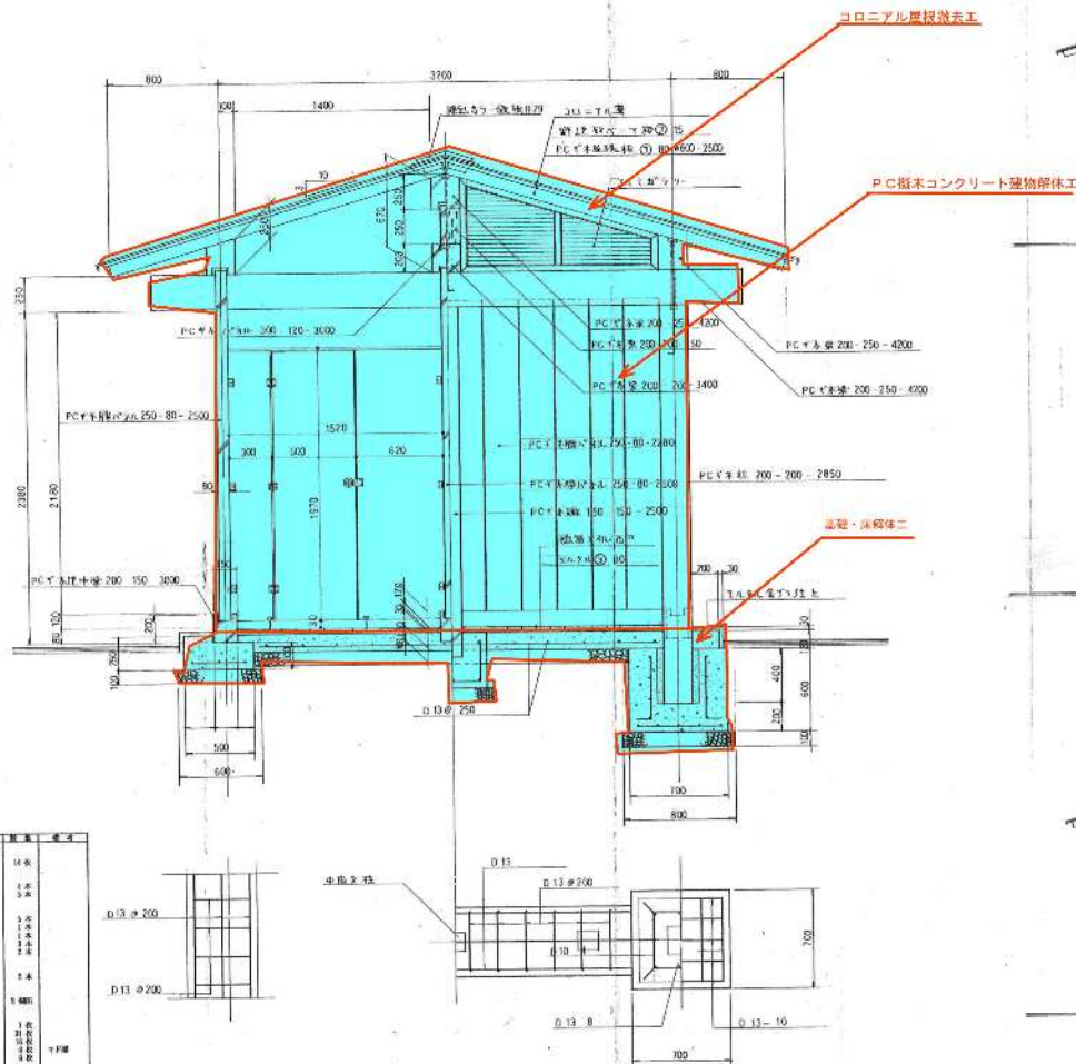
構造詳細図 S-1:20
