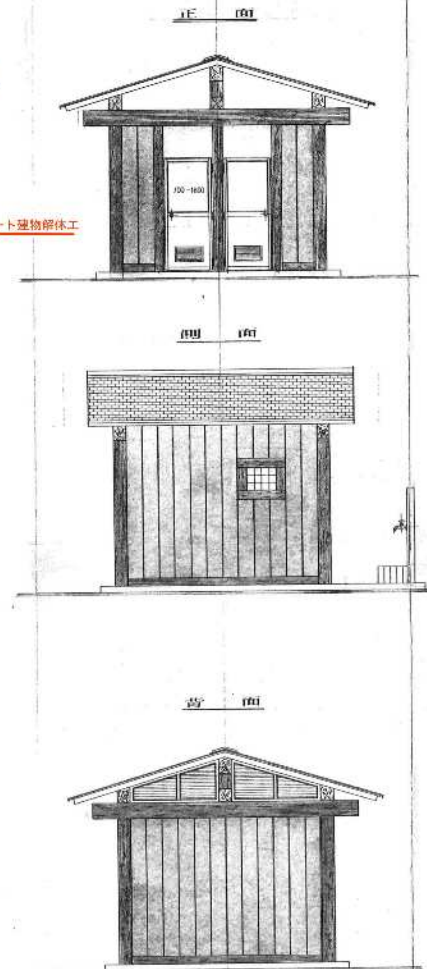
姿図 S-1:40
