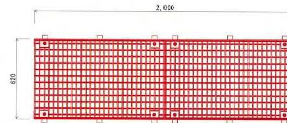
■製品平面図 ボルト固定タイプⅡ型(500用)
